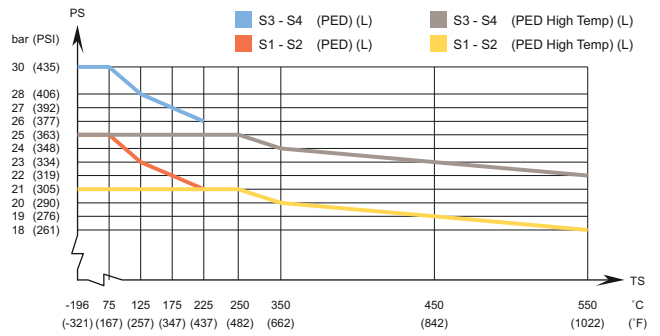
AlfaNova HP 27 - Gráfico de pressão/temperatura com aprovação do PED
