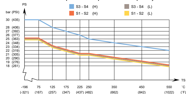
AlfaNova 27 - Gráfico de pressão/temperatura com aprovação do PED
