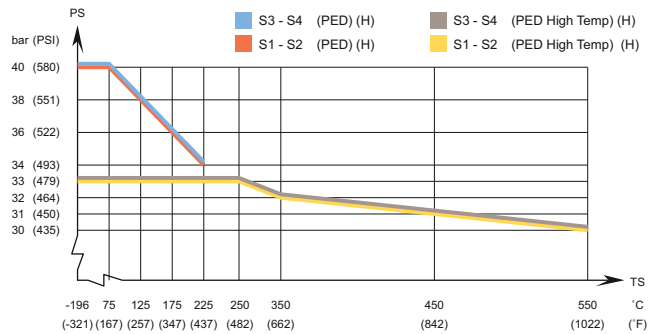
AlfaNova XP27 - Gráfico de pressão/temperatura com aprovação do PED
