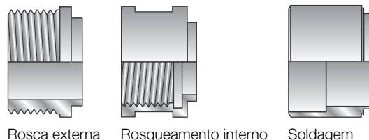
Rosca externa
